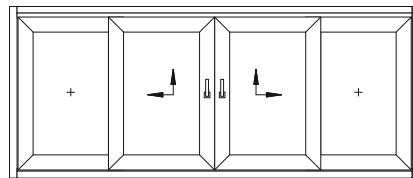
Schéma de ferrure C
