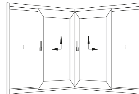
90°-Hoek als opening, twee bewegende vleugels, die naar buiten toe openen
