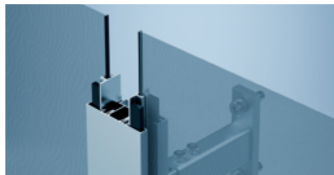
Centrale geleidingsrail heroal GR 37
